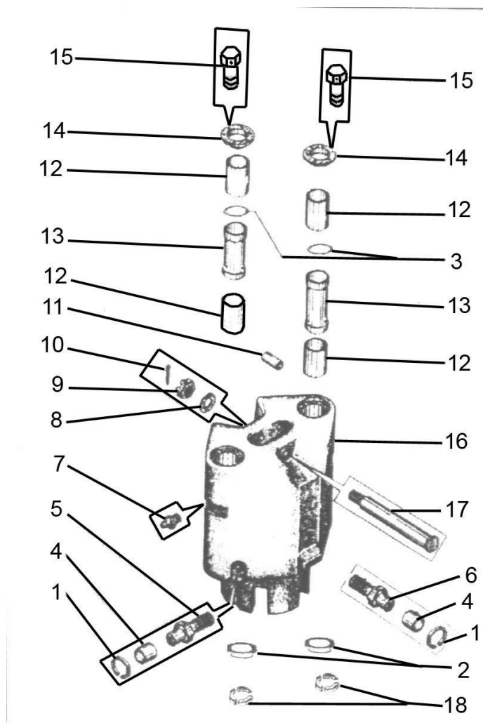
Рисунок 8- Цилиндр
