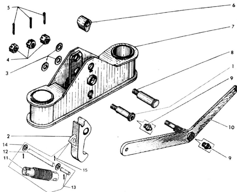
Рисунок 9- Кошка
