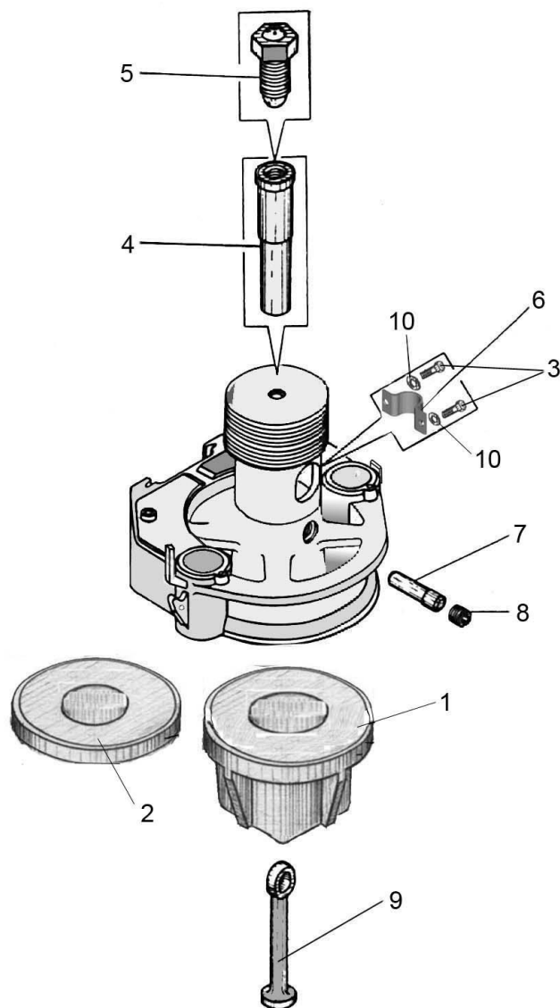
Рисунок 4- Блок поршня в сборе с наголовником
