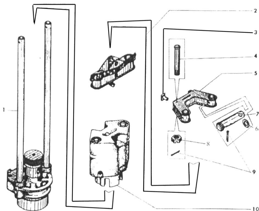
Рисунок 2- Составные части молота
