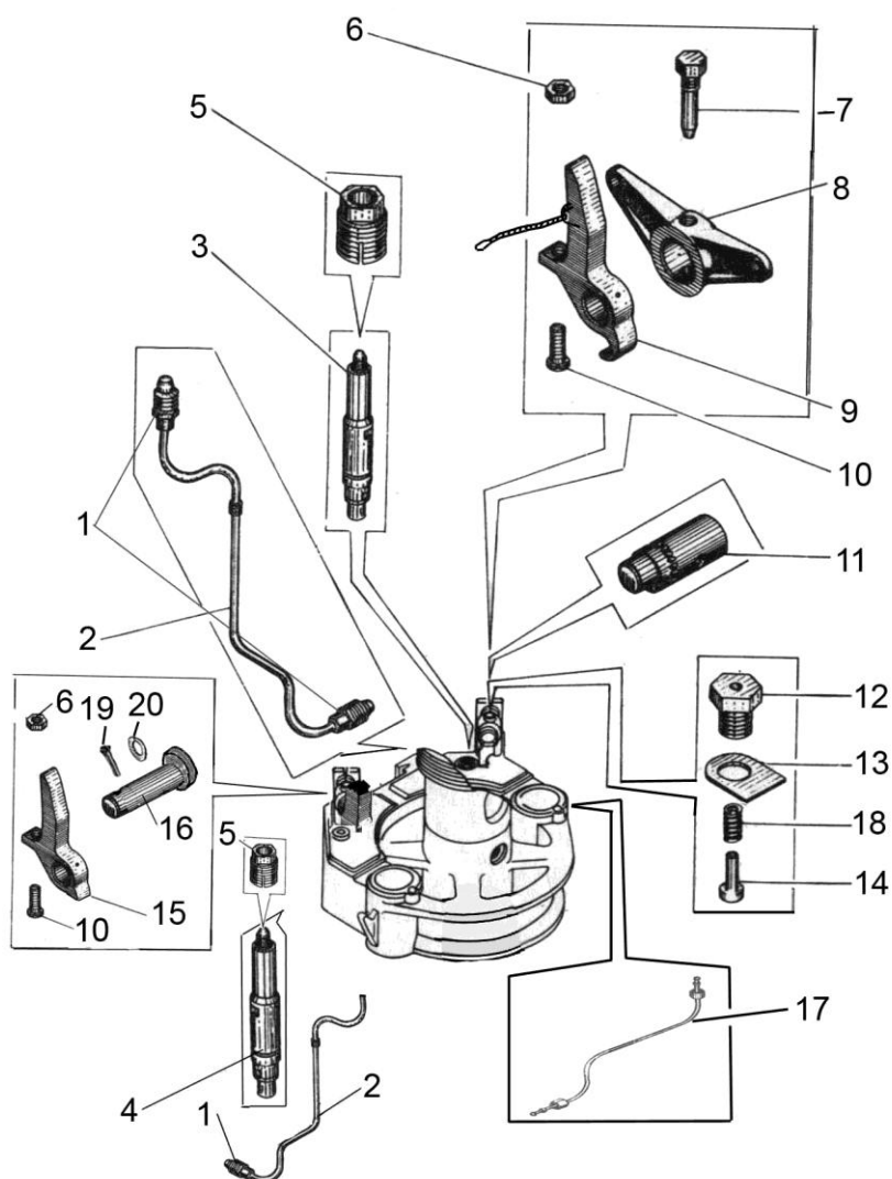
Рисунок 5- Блок поршня
