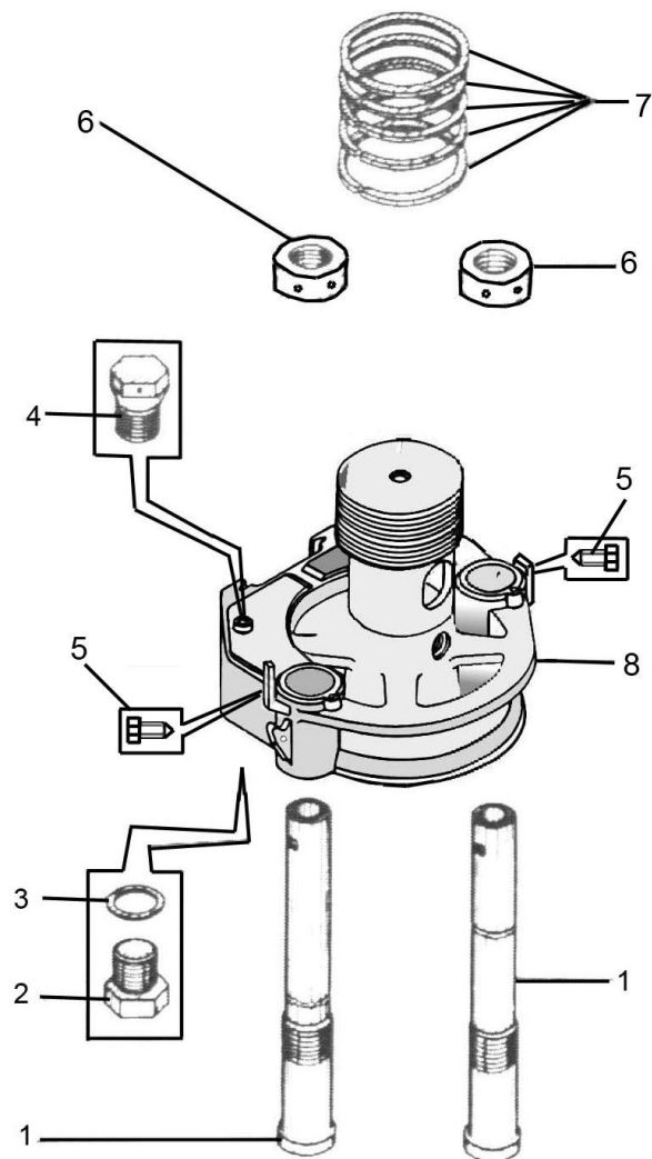
Рисунок 3- Блок поршня в сборе с штангами
