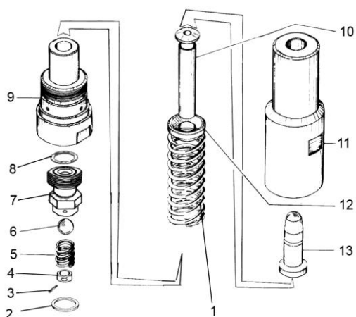
Рисунок 7а- Насос масляный
