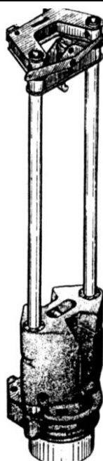
Рисунок 1- Общий вид молота
