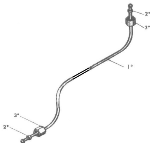
Рисунок 6- Маслопровод. Топливопровод
