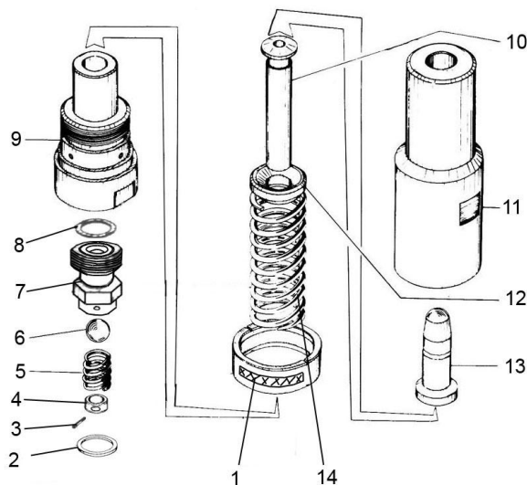
Рисунок 7- Насос топливный
