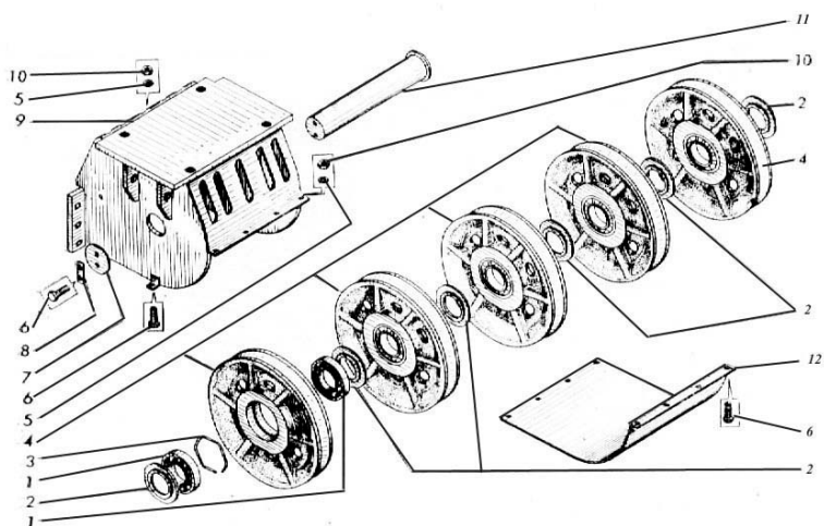
Рисунок 23- Обойма нижняя
