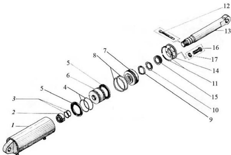
Рисунок 29- Гидроцилиндр выдвижения стрелки
