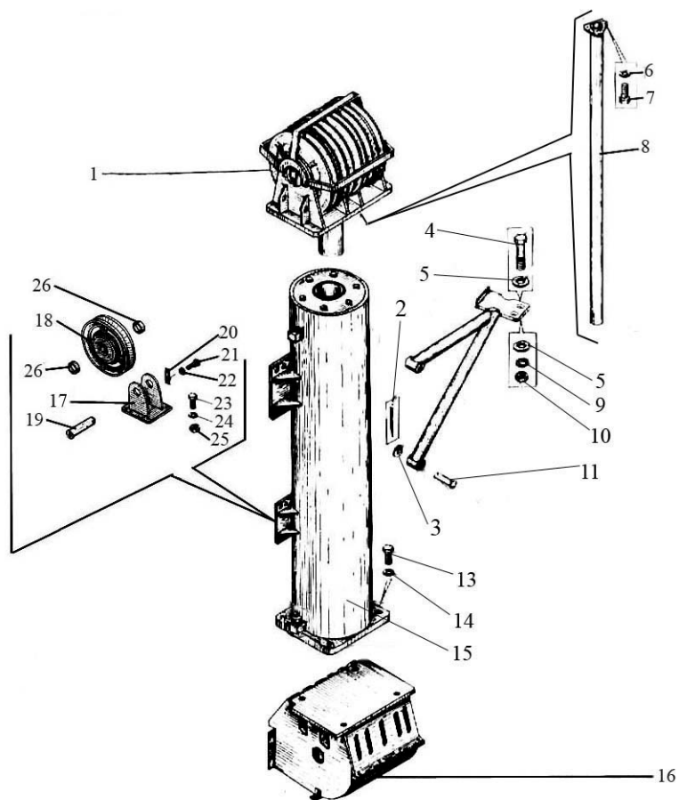
Рисунок 21- Полиспаст подъяема сваи
